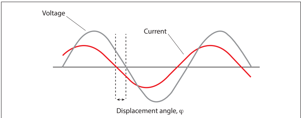
Fig. 7.1 Linear Load
