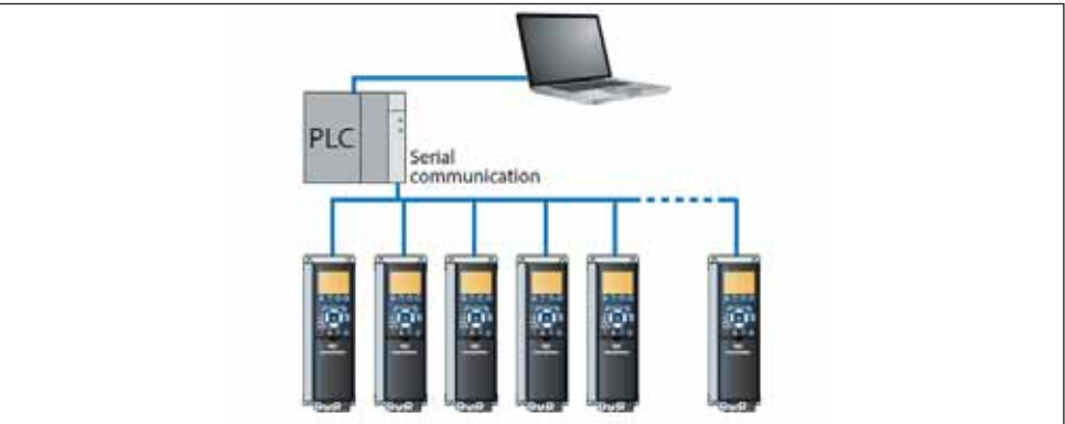
Fig. 8.8 Fieldbus wiring
