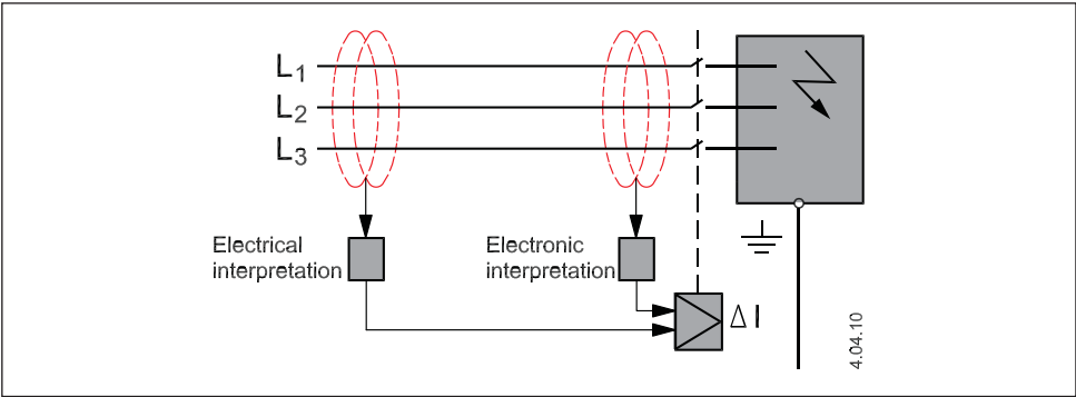
Fig. 6.8 Universal RCCB
